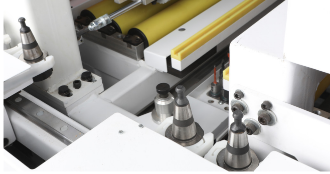
3+1 OTOMATİK TAKIM DEĞİŞTİRME ÖZELLİĞİ (ATC) 3+1 AUTOMATIC TOOL CHANGE (ATC) FEATURE
